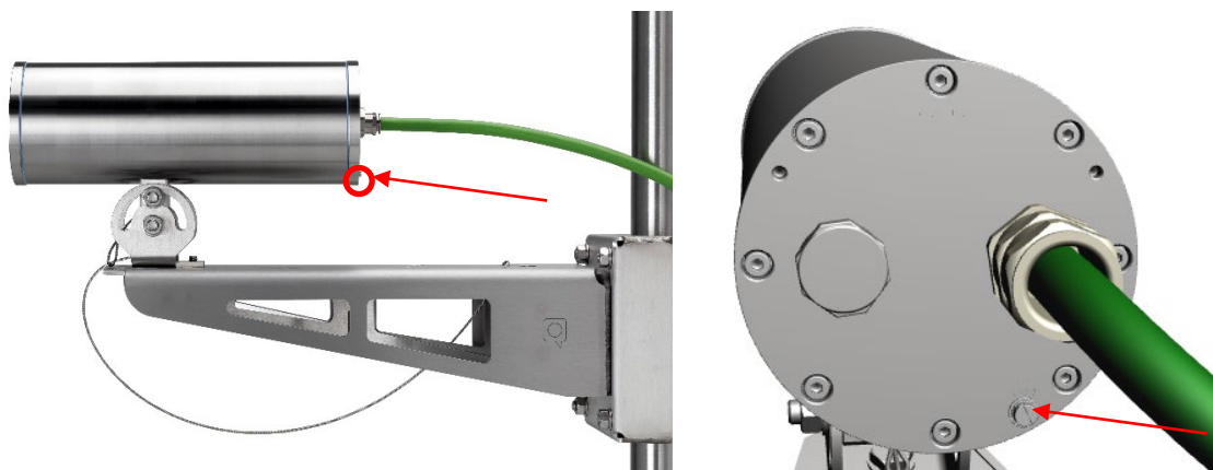
Fig. 5-1 RoughCam IPQ1656 Equipotential Bonding
